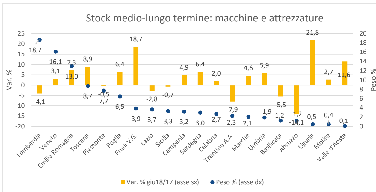
Figura 9 - Dinamica (giugno 18/17) dello stock di prestiti in bonis oltre il breve termine al settore agricolo per acquisto di macchine e attrezzature per regione e incidenza regionale sullo stock nazionale
