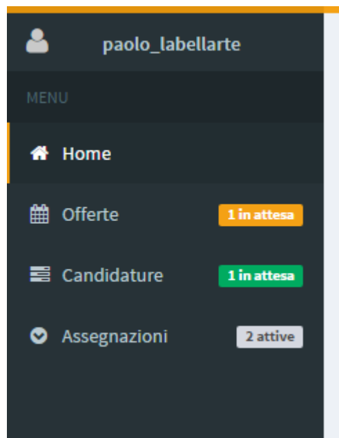
Figura 5 - menu
